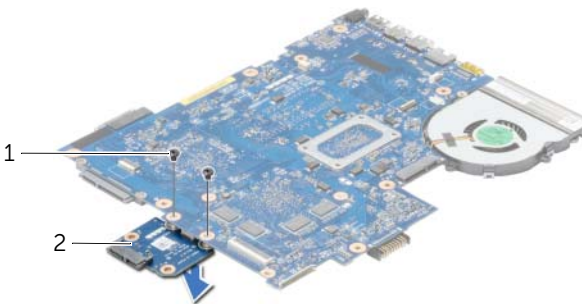
1 Schrauben (2) 2 Zwischenplatine des Festplattenlaufwerks
