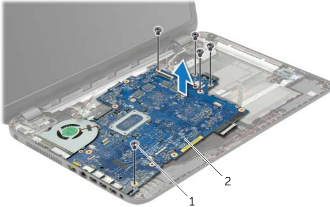
1 Schrauben (5) 2 Systemplatinenbaugruppe
